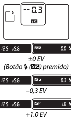
Disco de controlo secundário
