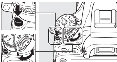
Disco dos modos de obturação
